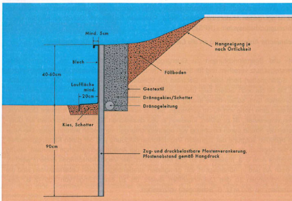
Bild 6.4_a und b: Prinzipskizzen Sperr- und Leiteinrichtungen für Amphibien. Eine Absturzsicherung ist erforderlich. Die Anwendung der „Richtlinien für passiven Schutz an Straßen durch Fahrzeugrückhaltesysteme (RPS)“ ist im Einzelfall zu prüfen.
