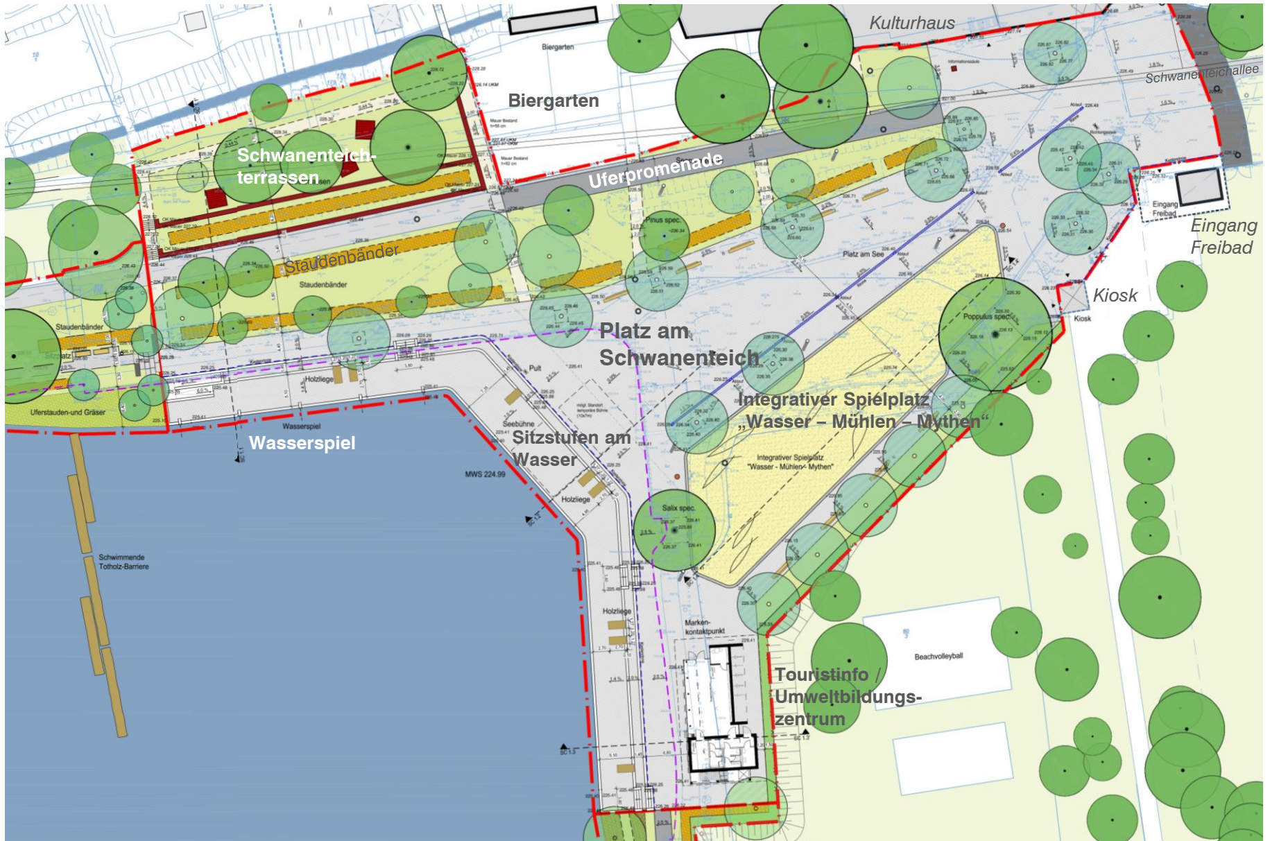
Entwurfsplanung 1. Bauabschnitt: Platz am Schwanenteich
